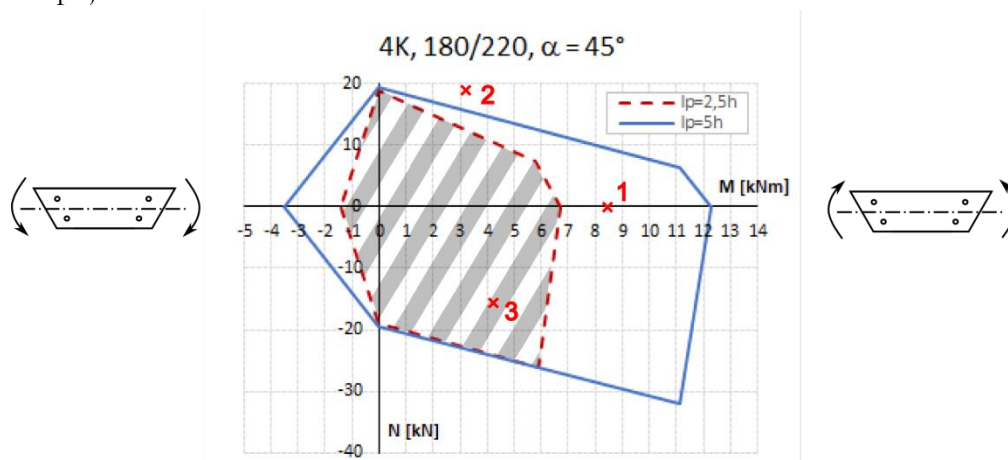
Obr. 8 Příklady užití návrhového diagramu M - N ; bod 1 odpovídá stropnímu trámu s převažujícím namáháním ohybovým momentem (vyboruje spoj s délkou L_p větší než 2,5b ), bod 2 představuje prvek namáháný především tahem a je mimo návrhové diagramy (plát by selhal), bod 3 ilustruje kombinované namáhání prvku vyskytující se např. u krokví (lze použít spoj minimální délky 2,5b s dostatečnou bezpečností). Levá část grafu se záporným ohybovým momentem ukazuje ohýbání spoje na nevhodnou stranu.
