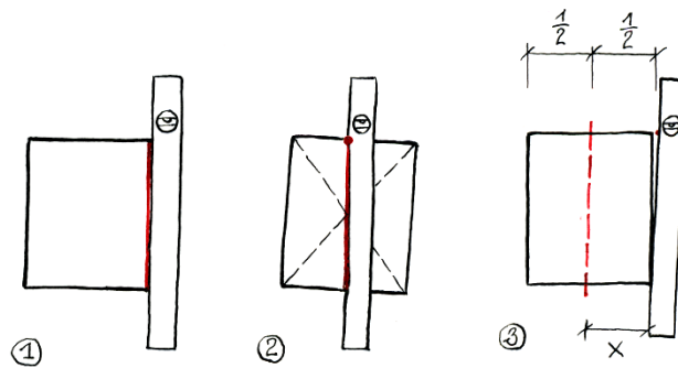
Obr. 17 Přesná metoda rozměření profilu trámu; 1 - určení sklonu ve středu zamyšleného trámu, 2 – vynesení osy řezu na odříznutém čele, 3 – určení polohy bodu druhého dělicího bodu na konci plátu
