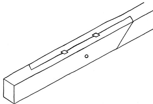
Obr. 36 Plátovaný spoj po sesazení a zajištění
