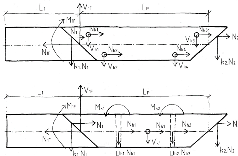
Obr. 7 Síly působící v plátu se čtyřmi kolíky (nahoře) a v plátu s dvěma hmoždíky a jedním kolíkem (dole).
