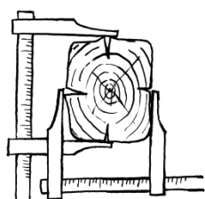
Obr. 13 Zohlednění deformací při měření profilu
