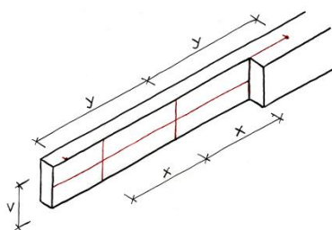
Obr. 24 Rozměření délky plátu
