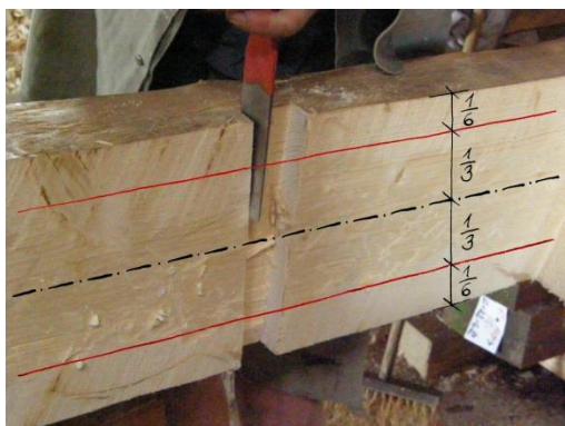
Obr. 31 Podebrání dvou třetin vnitřní středové části plátu, styčné plochy zůstávají pouze po okraji plátu
