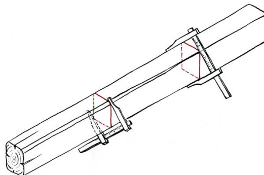
Obr. 11 Měření minimálního průměru kulatiny v místě oblin
