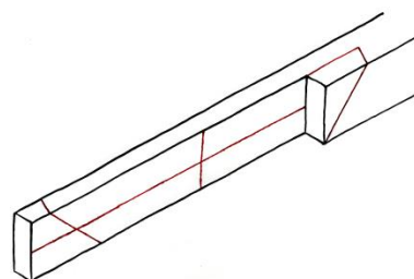
Obr. 26 Vynesení rysek šikmého podkoseného čela
