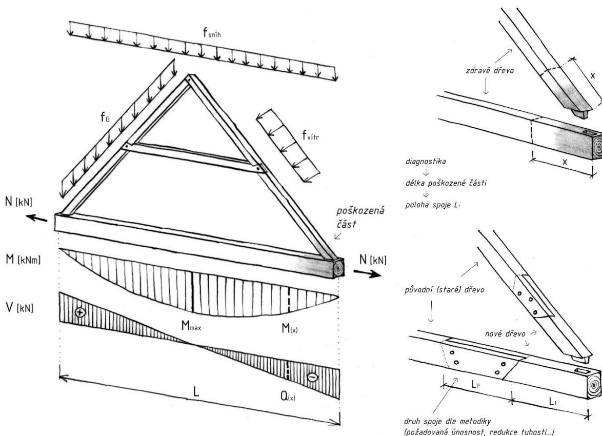
Obr. 1 Vazba s poškozenými prvky a průběh opravy
