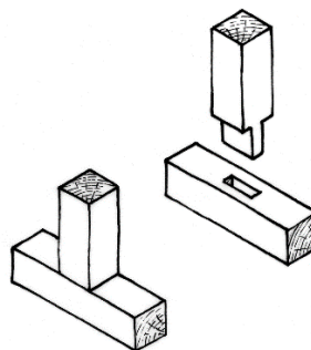
Obr. 3 Čep a dlab [2]
