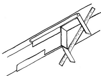
Obr. 25 Vynesení rysek příčného řezu čel plátu
