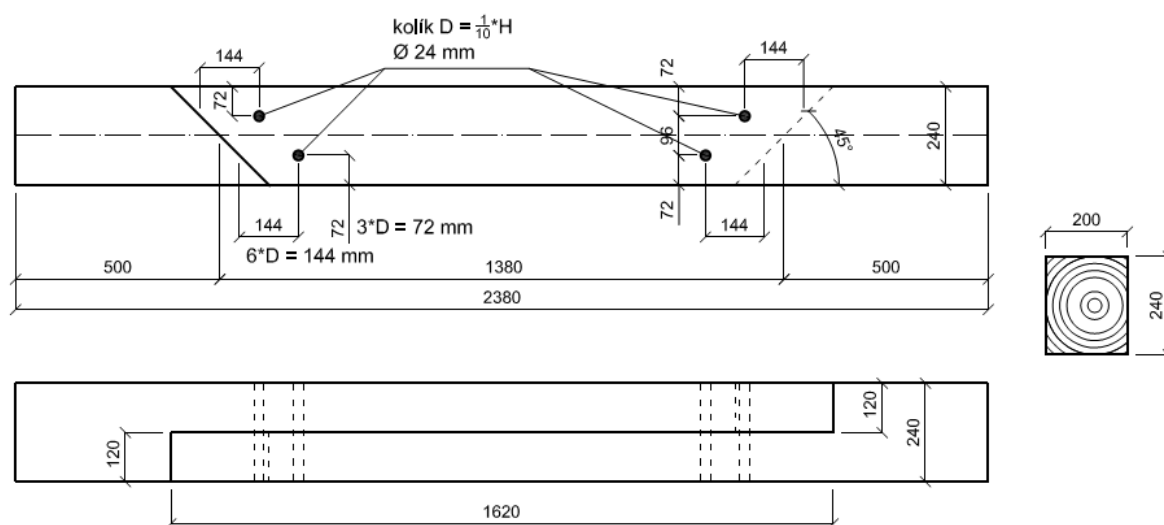
Obr. 1: Rozměry tesařského spoje
