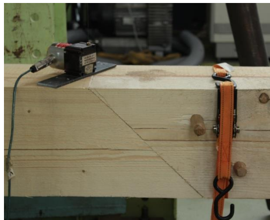
Obr. 2: a) Připravený spoje před experimentem – zkouškou v třibodovém ohybu; b) detail šikmého čela a dvou dřevěných kolíků
