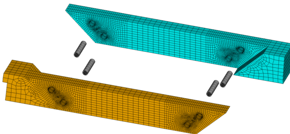
Obr. 3: Výpočtový numerický model tesařského spoje vytvořený v programu ANSYS
