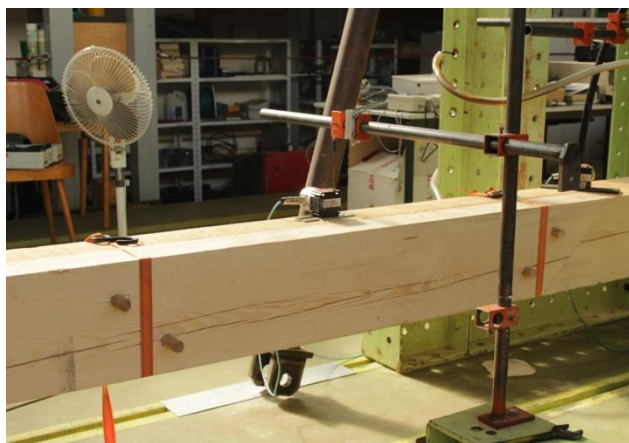
Obr. 2: a) Připravený spoje před experimentem – zkouškou v třibodovém ohybu; b) detail šikmého čela a dvou dřevěných kolíků
